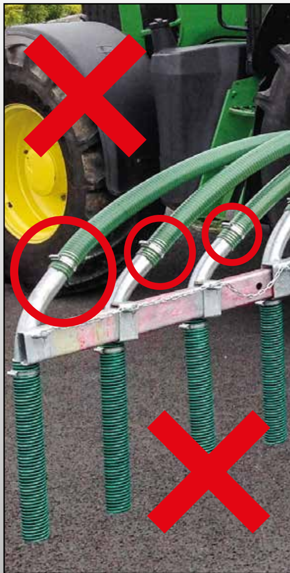
50 mm slanger m/ innvendige stålrør som gir blokkeringer.
