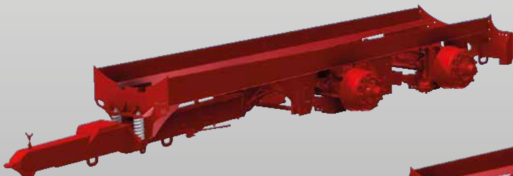
SlurryKats utprøvde og unike pressformede og koniske chassis komplett med 6-punks montert hjuloppheng
