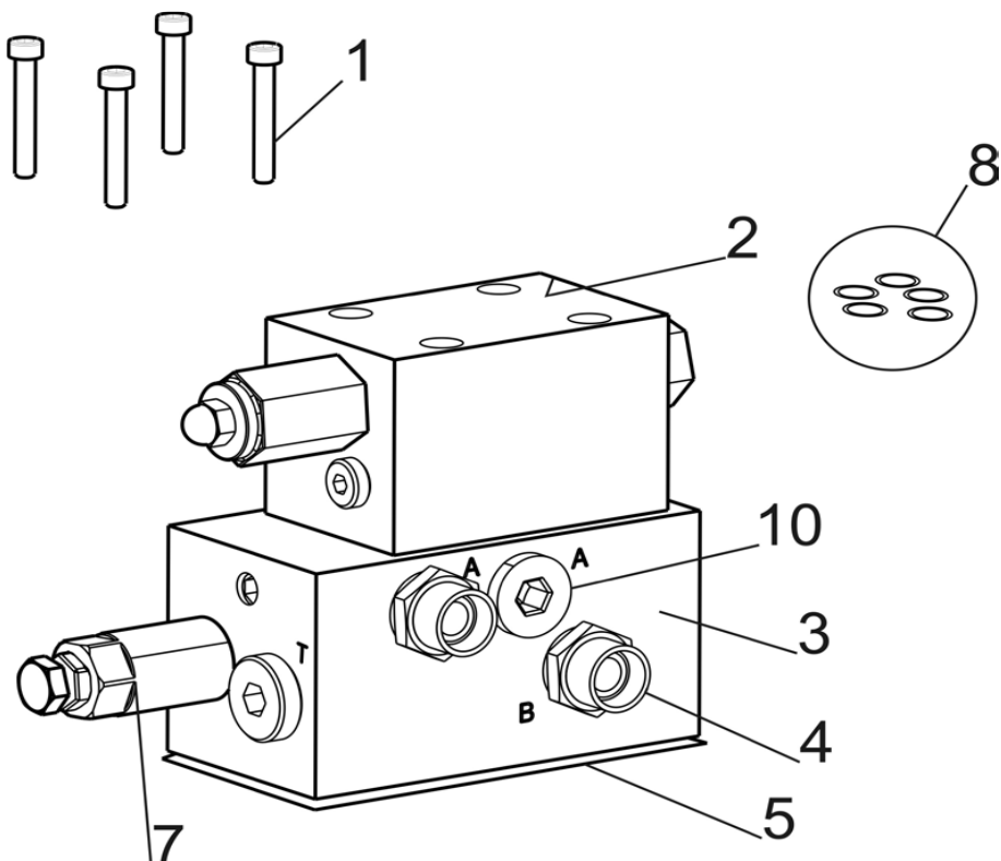
Riktningsventil
