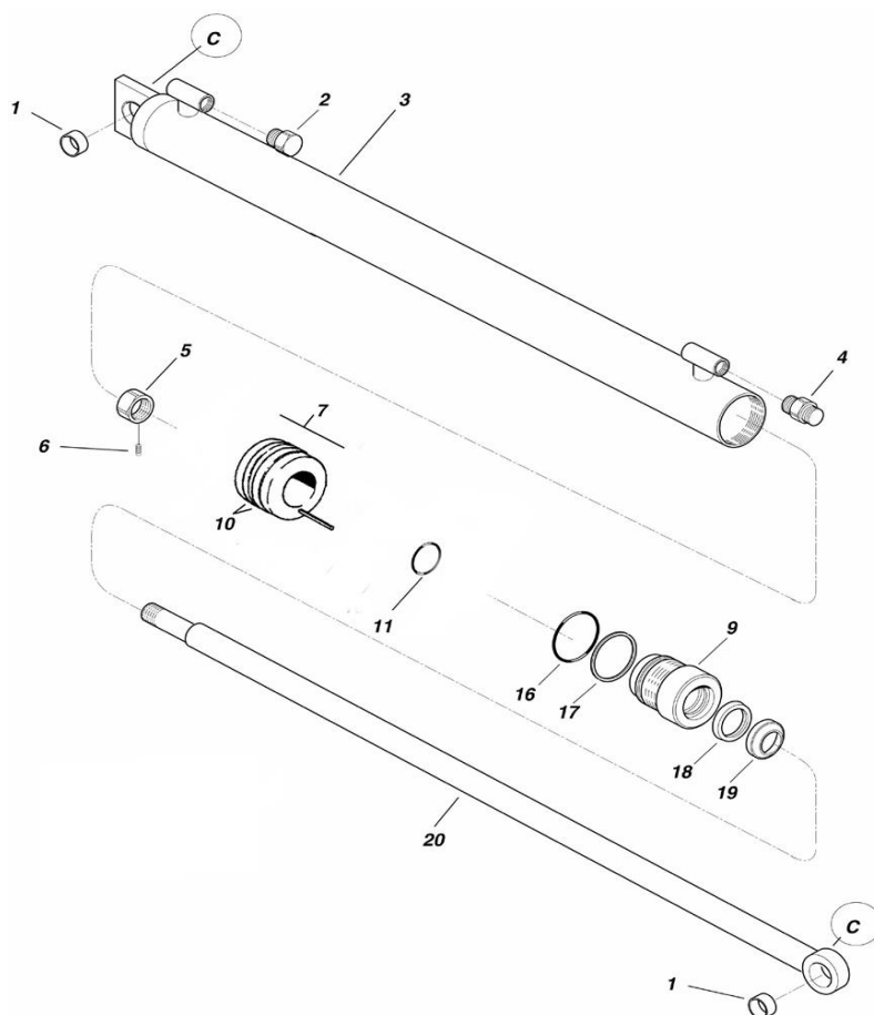
Cylinder 45/30 x 480 med C/V
