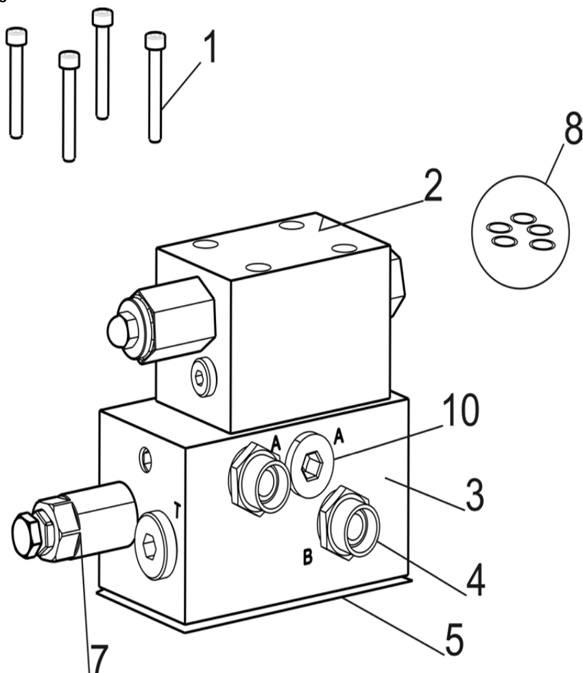
Riktningsventil
