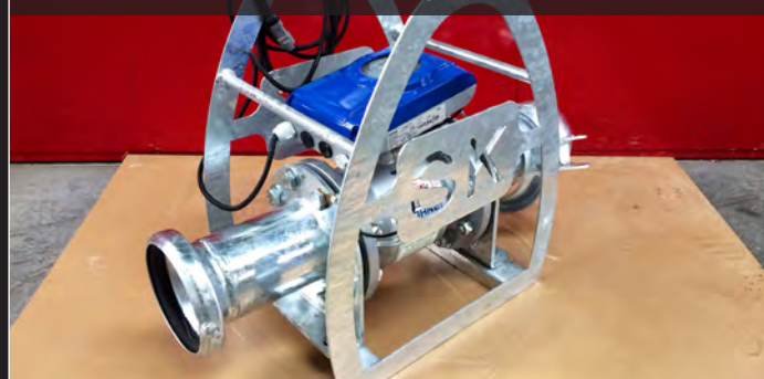
Flowmeter montert i galvanisert stativ
